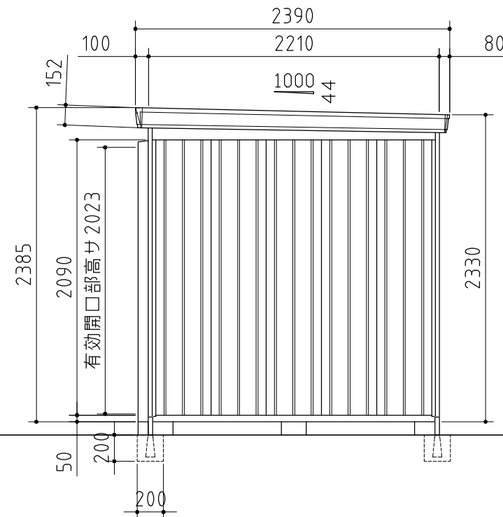
側面図
